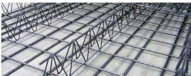
KIMMU® Hy Rib
